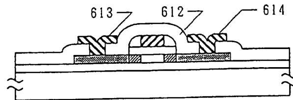
Fig. 6F Prior Art
